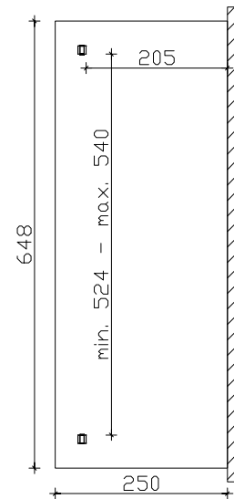
Grundriss
