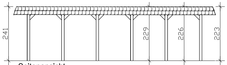
Seitenansicht
