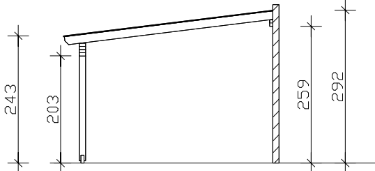
Seitenansicht
