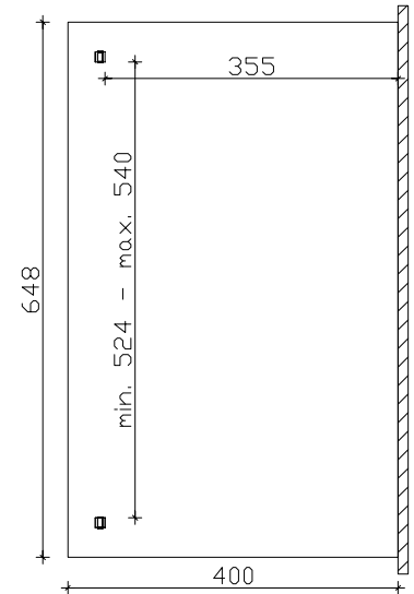
Grundriss
